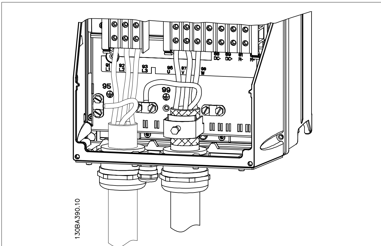
Ilustracja 5.22: W pierwszej kolejności zakończyć uziemienie silnika, następnie umieścić przewody silnika U, V i W w zacisku i dokręcić. Sprawdzić, czy zewnętrzna izolacja kabla silnikowego została usunięta z zacisku EMC.
