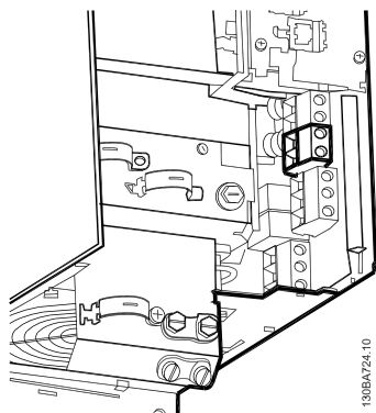
Ilustracja 5.29: Zacisk podłączenia rezystora hamowania dla B3.
